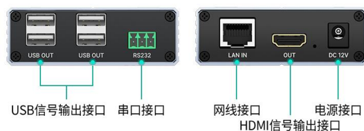
接收器RX
