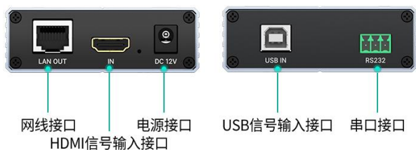
发射器TX
