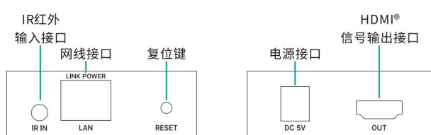
接收器
