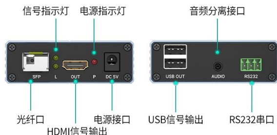
接收器RX
