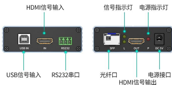
发射器TX
