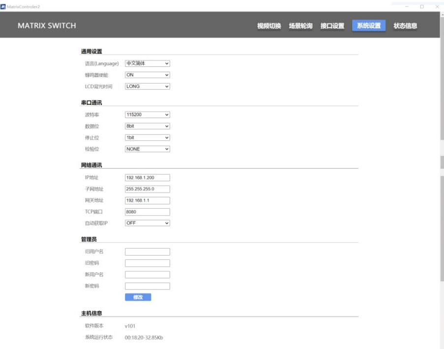
图7：系统设置界面
